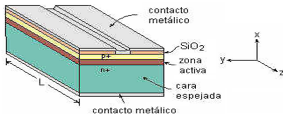
Fig. 3. Estructura láser semiconductor
