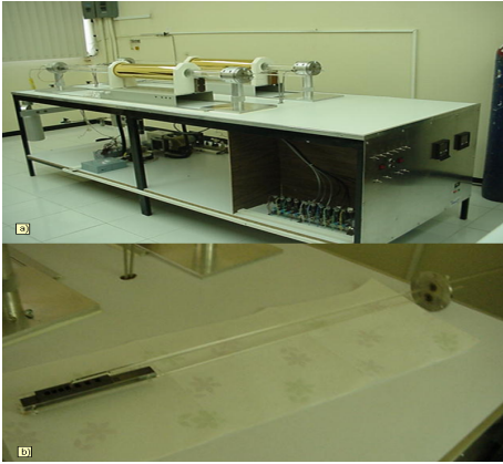
Fig. 6. a) Sistema de epitaxia desde Fase Líquida diseñado y construido en el CIDS-ICUAP. b) Vista del bote deslizante (sliding) y su manipulador en su soporte de cuarzo. (cortesía BUAP) [5]
