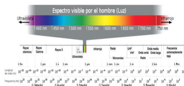
Figura 1. Espectro electromagnético [2]
