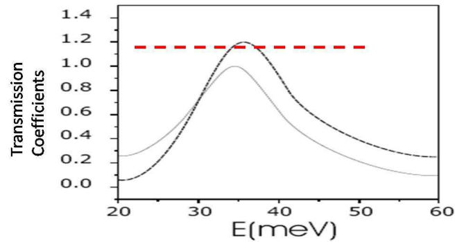
Fig. 4 Coeficientes de transmisión superiores a la unidad para valores grandes de la magnitud que caracteriza la mezcla de huecos. A.D. Snchez y C.R. Poetto, J. Phys., Condens., Matter 7, 2059 (1995).
